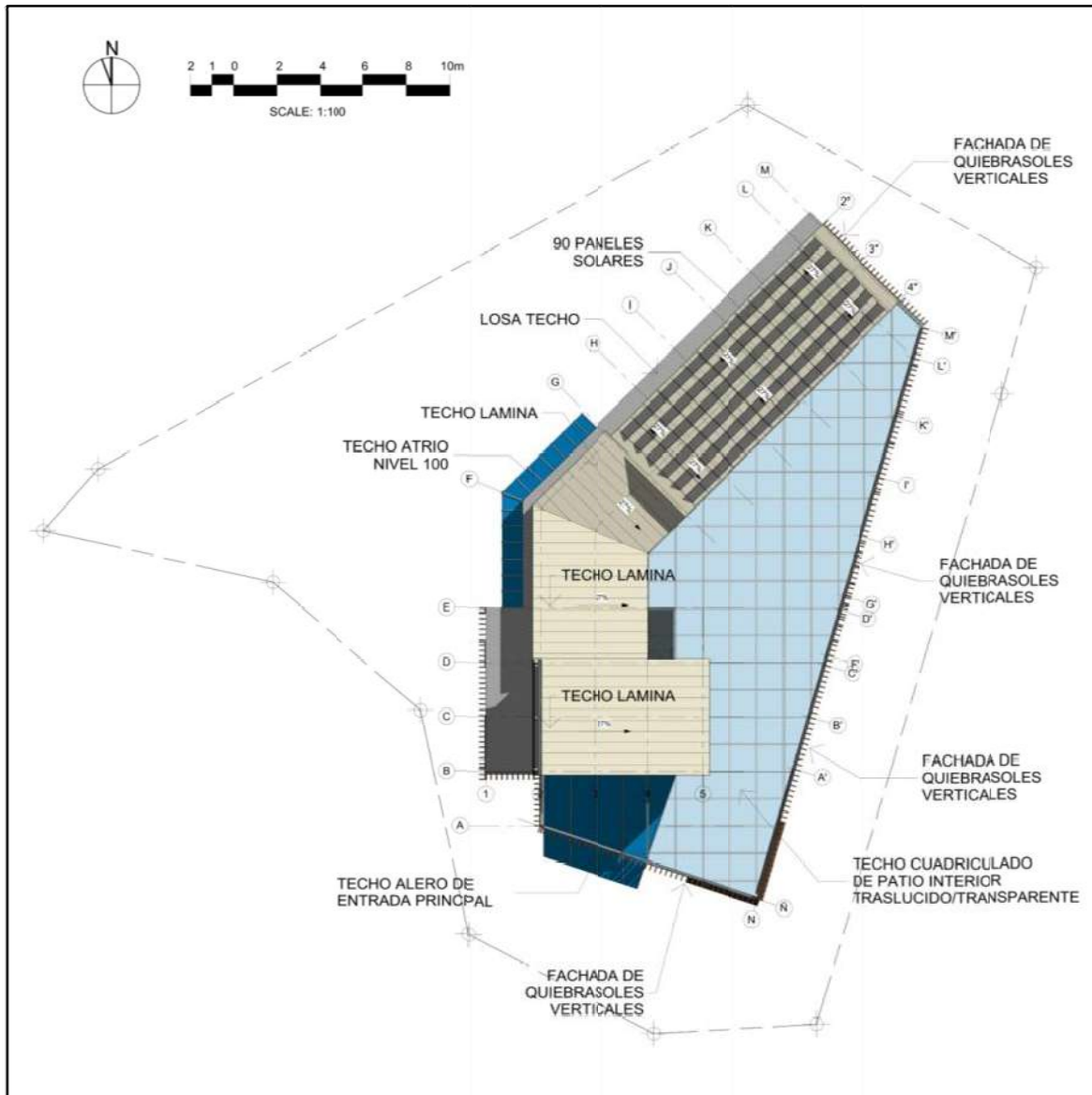
Ilustración 86-Planta de techo
