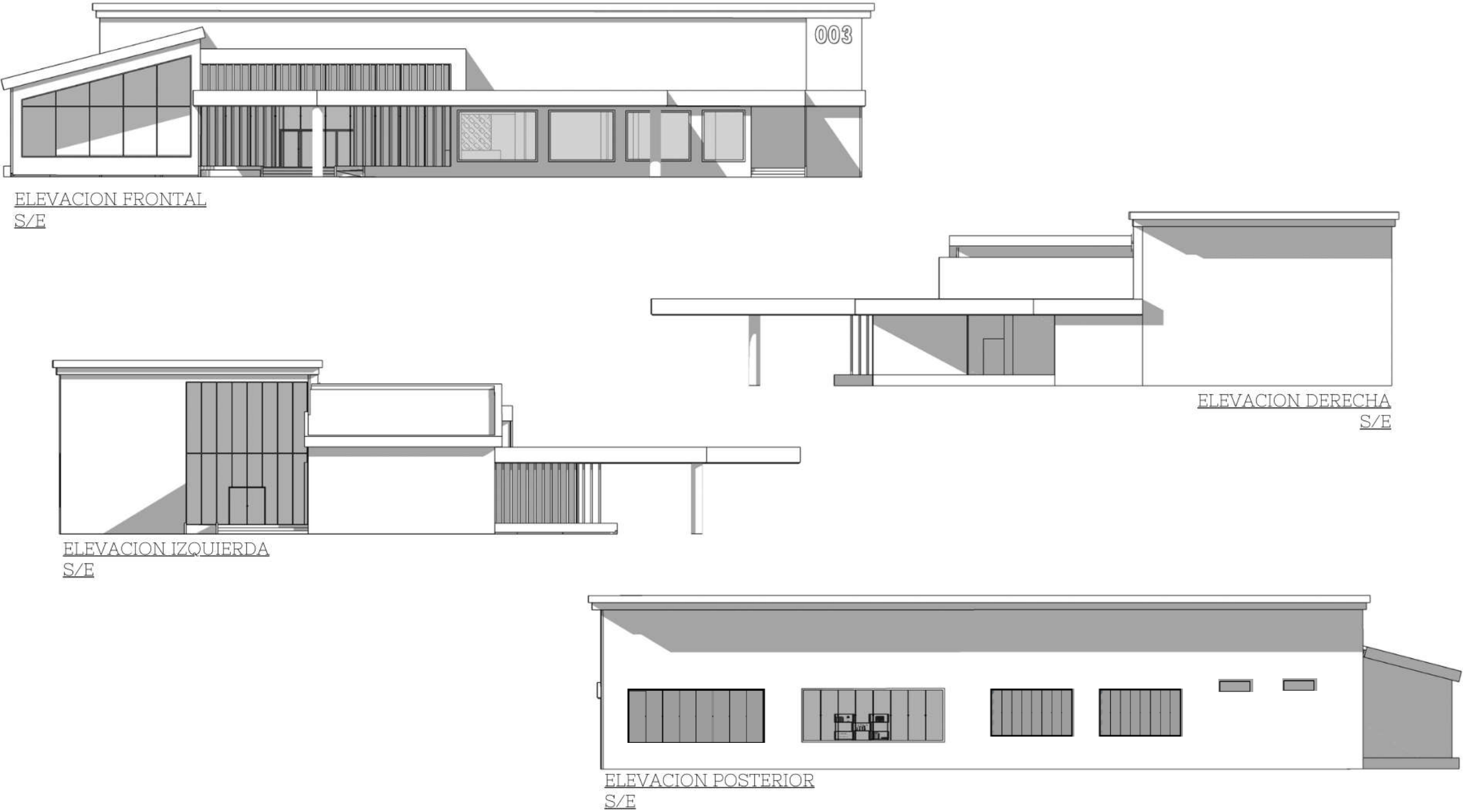
Ilustración 39 Elevación de edificio 003 Administración y Cultura Nota. Realizado por Brenda González
