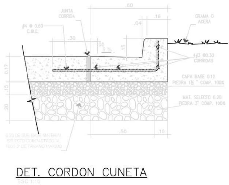
Ilustración 48 Detalle Cordón Cuneta
