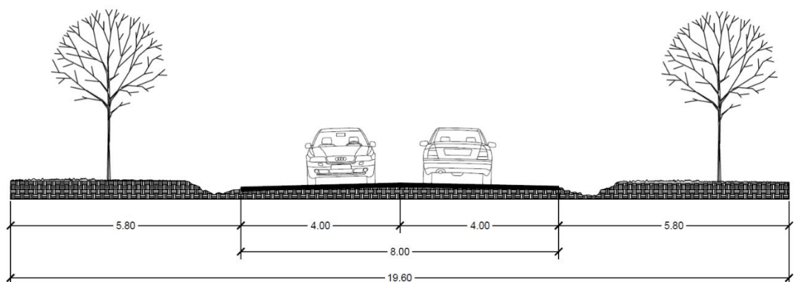
Gráfico 8. (Sección de la vía principal, Ave. Belisario Porras) Fuente: Propiedad de Mariaesther Vigil M. (3 de abril de 2022).
