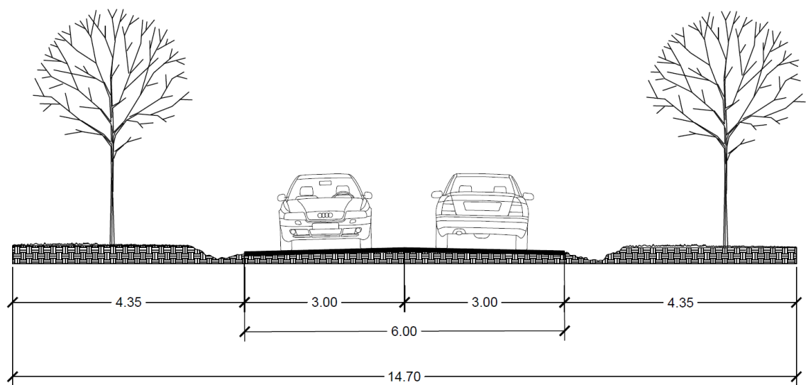
Gráfico 9. (Sección de las vías secundarias, Carretera Órea, Vía El Sesteadero) Fuente: Propiedad de Mariaesther Vigil M. (3 de abril de 2022).
