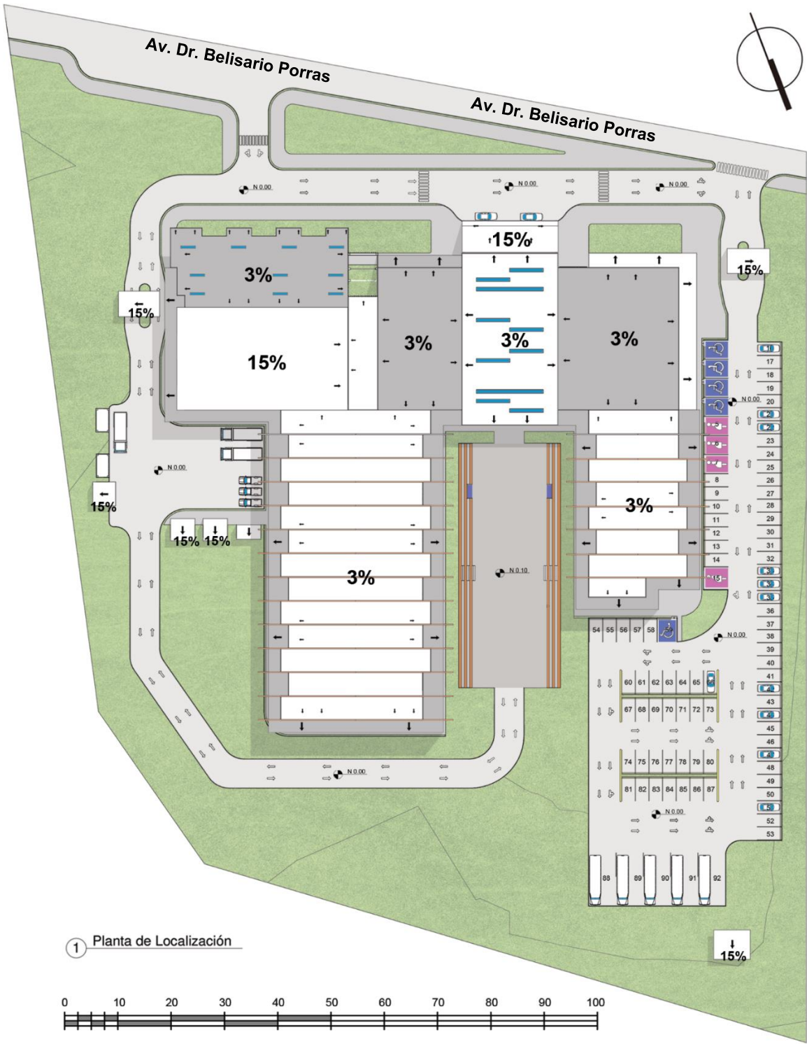
Plano 03 (Localización General)
