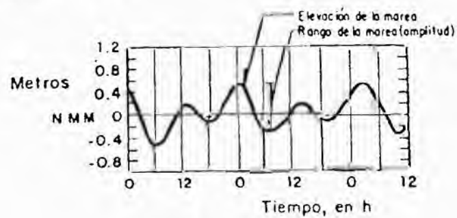
c) Mixta
