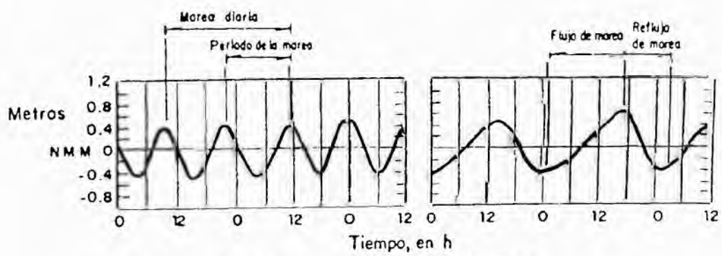
a) Semidiurna
