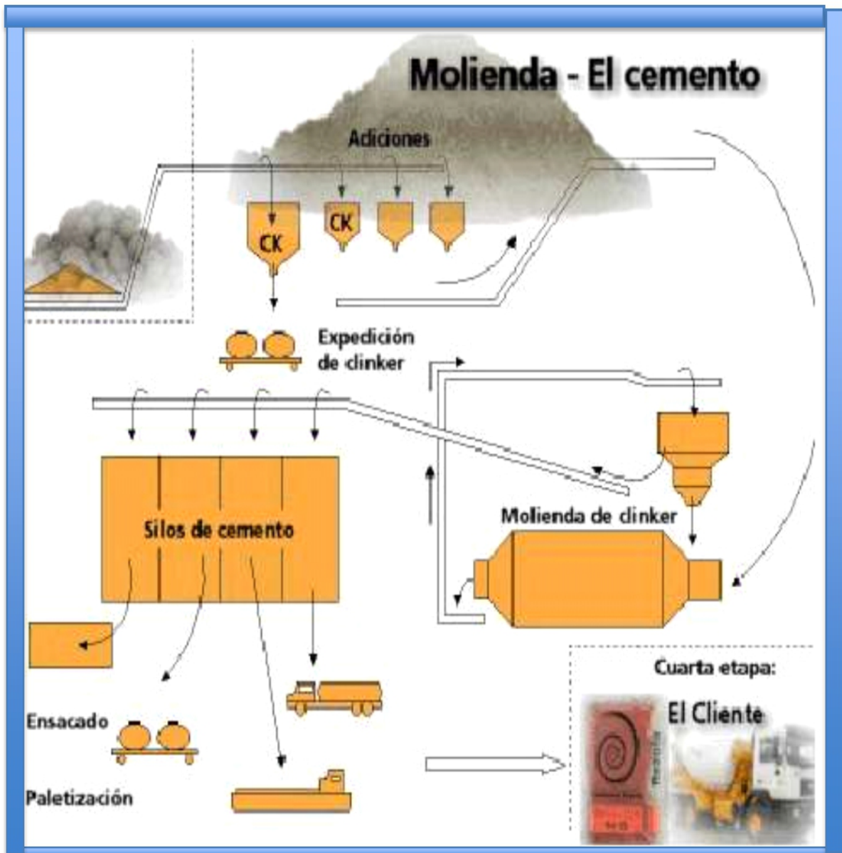
Imagen N° 22. Proceso de Molienda – El cemento.
