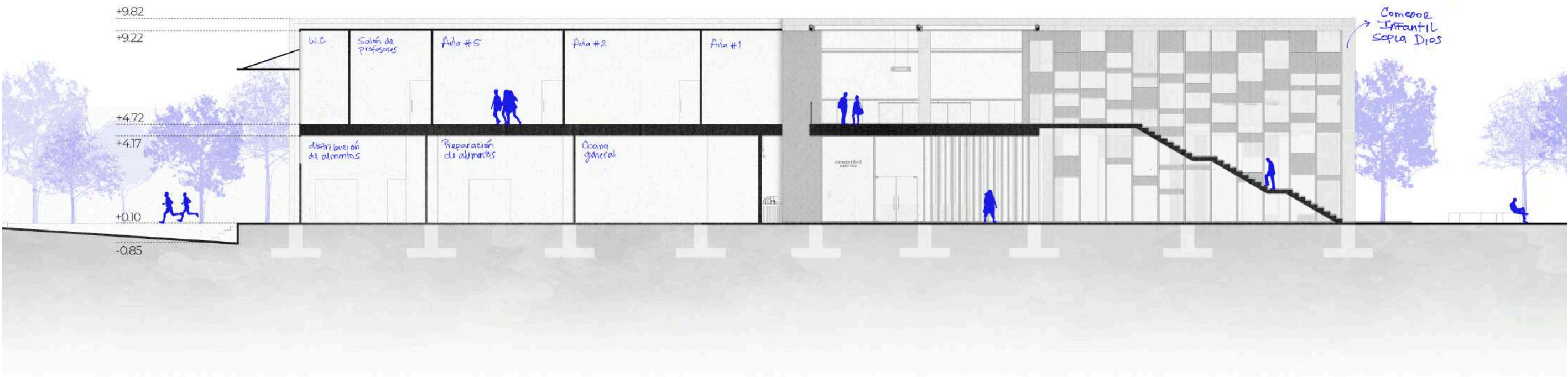
Figura 35. Sección transversal. Elaborado por el autor.
